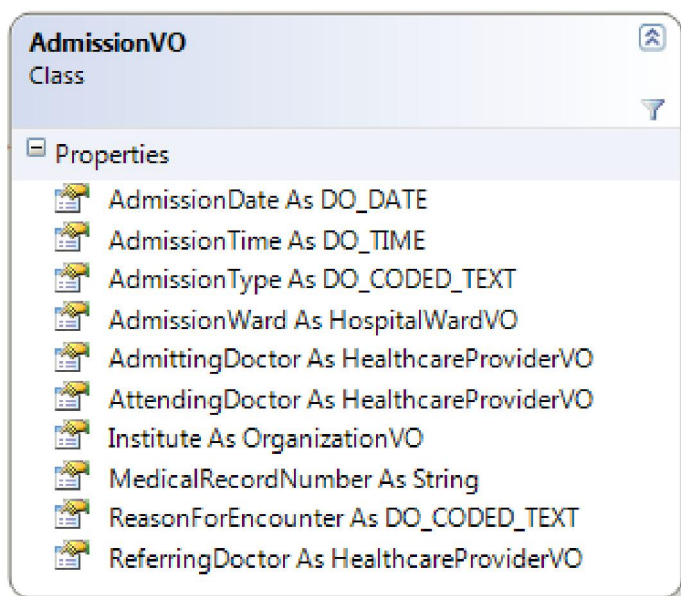
شکل ۴ - کلاس AdmissionVO
