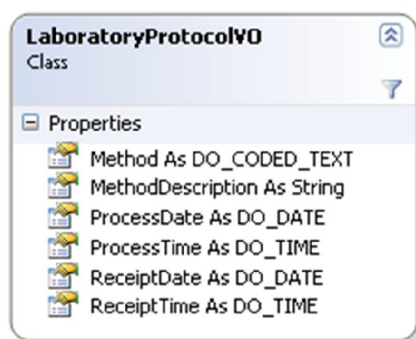
شکل ۱۴ - کلاس LaboratoryProtocolVO
