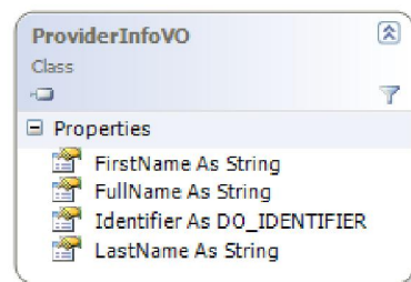
شکل ۶ - کلاس ProviderInfoVO
