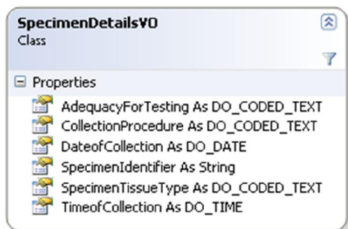
شکل ۱۳ - کلاس SpecimenDetailsVO
