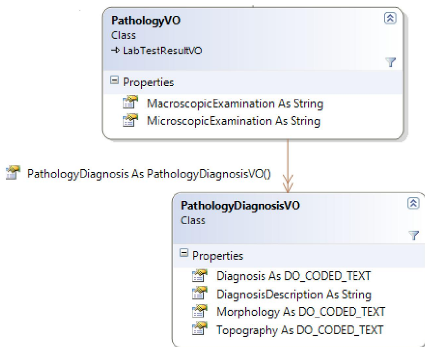
شکل ۱۱ - کلاس PathologyVO
