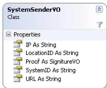
شکل ۱۷ - کلاس SystemSenderVO
