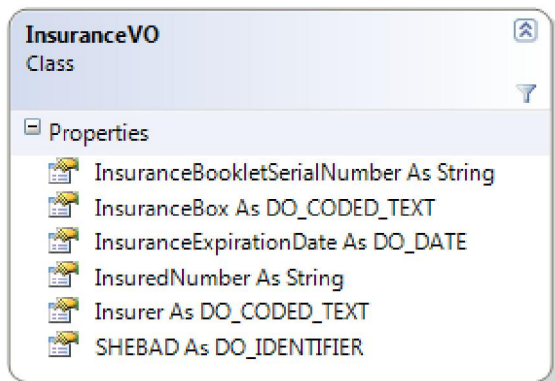
شکل ۷: - کلاس InsuranceVO
