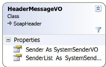
شکل ۱۶ - کلاس HeaderMessageVO
