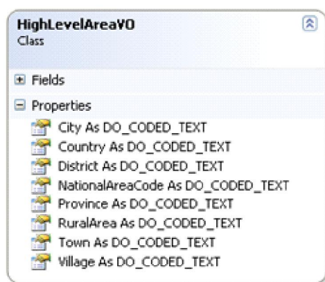
شکل ۹ - کلاس HighLevelAreaVO
