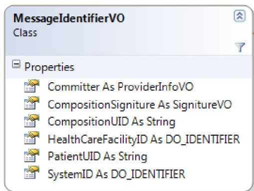
شکل ۱۵ - کلاس MessageIdentifierVO
