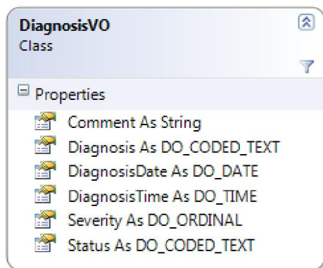
شکل ۱۲ - کلاس DiagnosisVO
