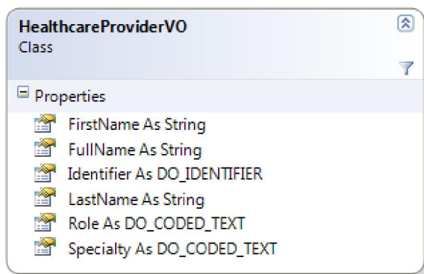
شکل ۵ - کلاس HealthcareProviderVO
